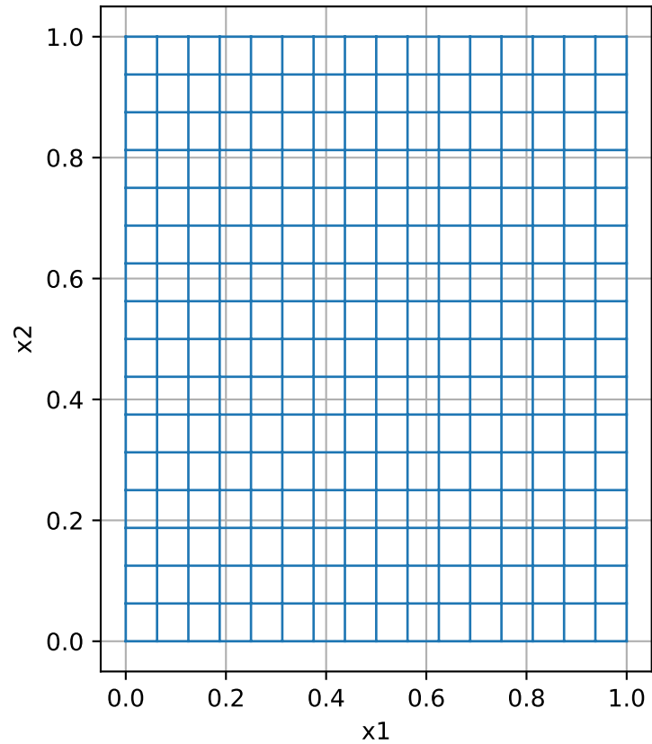
TensorMesh
